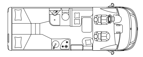
ECOVIP H2109 INTEGRIERTER
