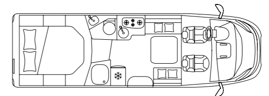
KOSMO EMBLEMA 512E
